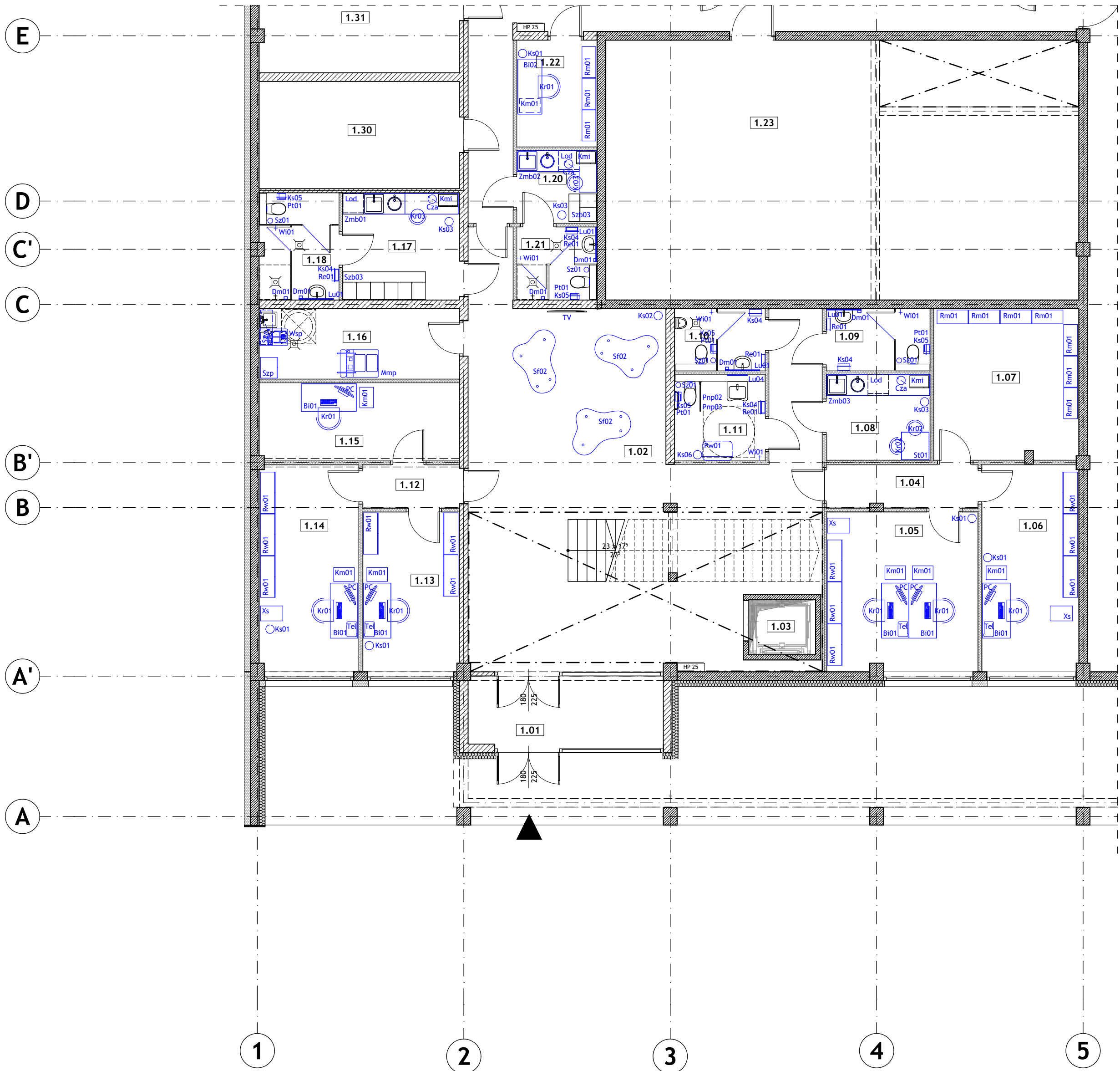
RZUT 0.PARTERU
