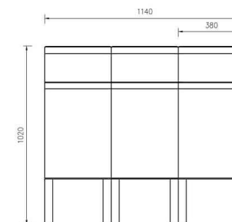
FRONT KOSZA
