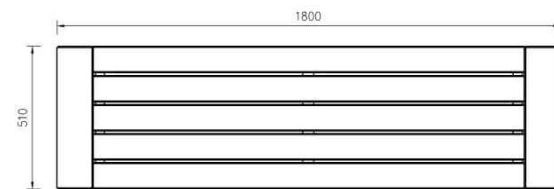
RZUT ŁAWKI
