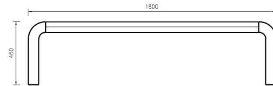
FRONT ŁAWKI
