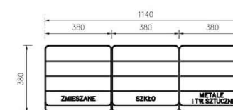
RZUT KOSZA
