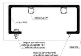
Szyina PEN
